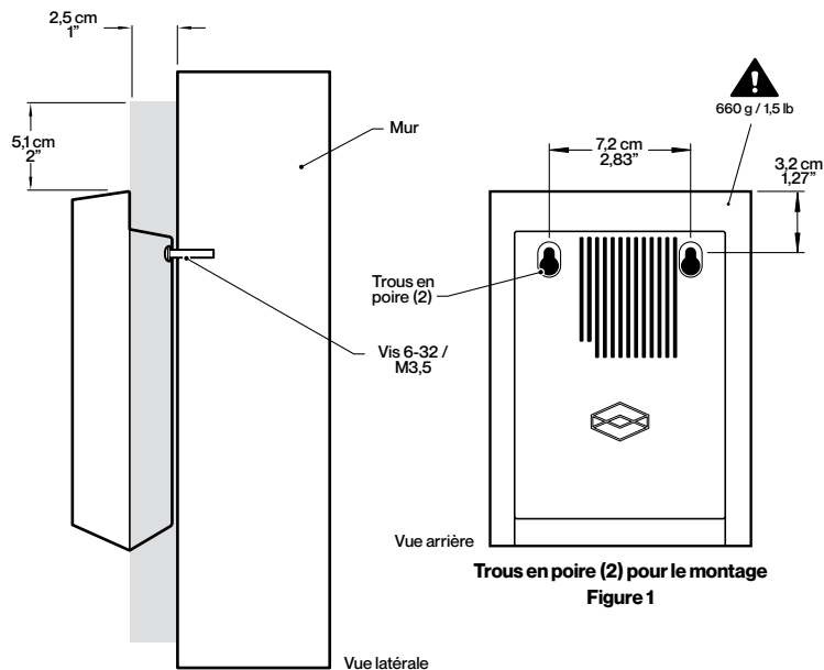
Ventilation - Dégagements pour la circulation de l'air Figure 2
