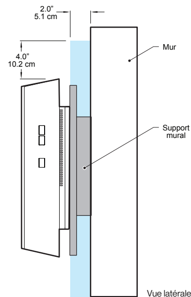
Ventilation - Dégagements pour la circulation de l'air Figure 2
