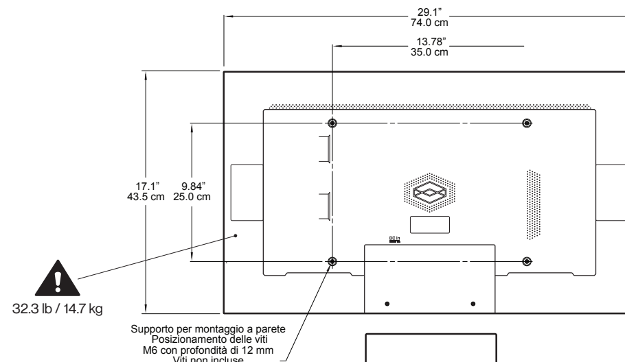
Inserti filettati (4) per il montaggio Figura 1
