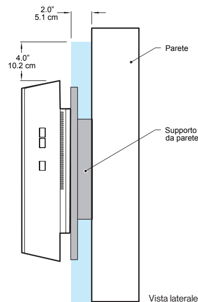
ziona - Spazi per la circolazione dell'aria Figura 2
