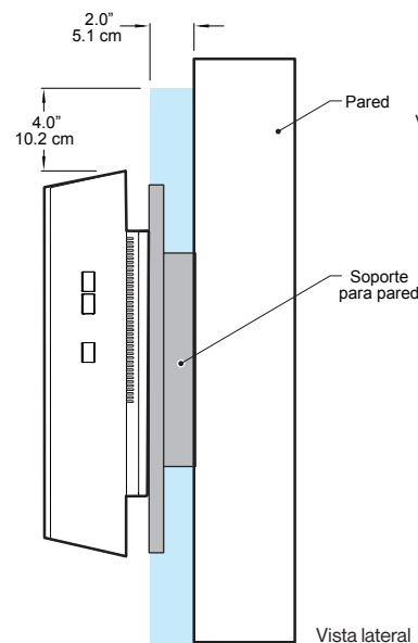
Ventilación - Espacios para el flujo de aire Figura 2
